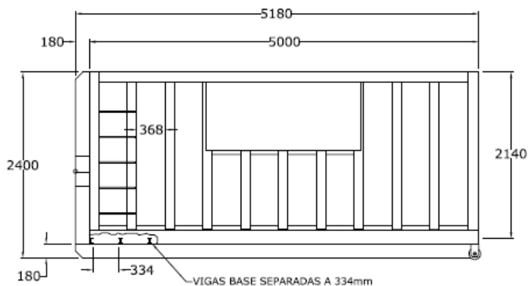
1 HOJA APERTURA BASCULANTE LATERAL
