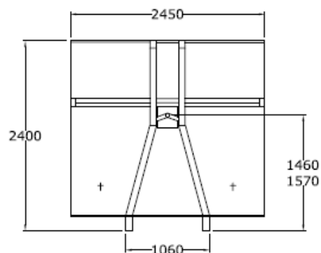
1 HOJA APERTURA LATERAL
